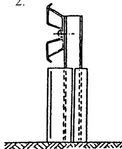
Załącznik 11.5. Dodatkowe urządzenia zabezpieczające użytkowników pojazdów jednośladowych na łukach drogi, wg [32]
