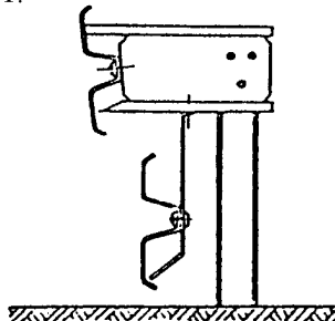
Załącznik 11.5. Dodatkowe urządzenia zabezpieczające użytkowników pojazdów jednośladowych na łukach drogi, wg [32]
