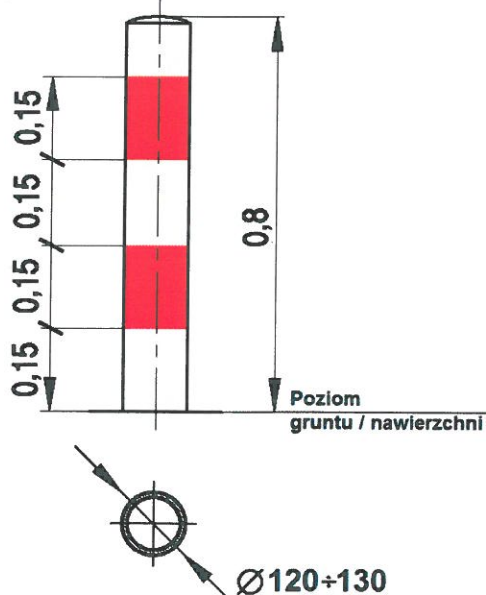
Rys. 1 - Zwymiarowany słupek po montażu
