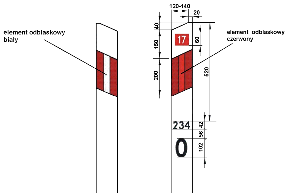
Rys.1. Słupek prowadzący U-1a z naniesionym numerem drogi, znakiem kilometrowym i hektometrym, przeznaczony do umieszczenia na poboczu drogi, w hektometrze zerowym
